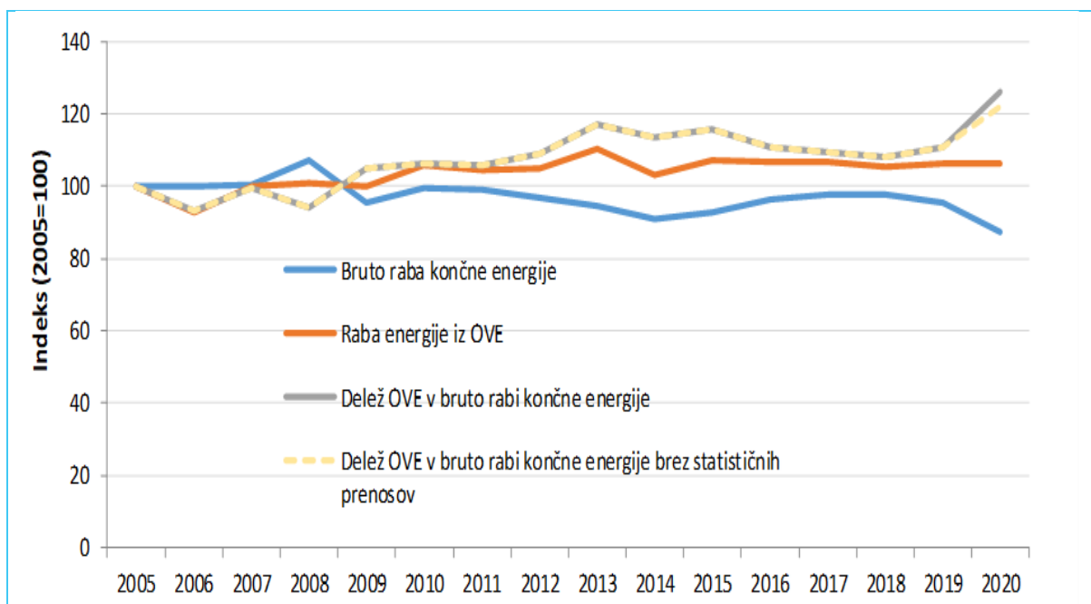
Slika 26: Gibanje bruto rabe končne energije, rabe OVE in deleža OVE glede na leto 2005 (Vir: SURS, IJS-CEU)
