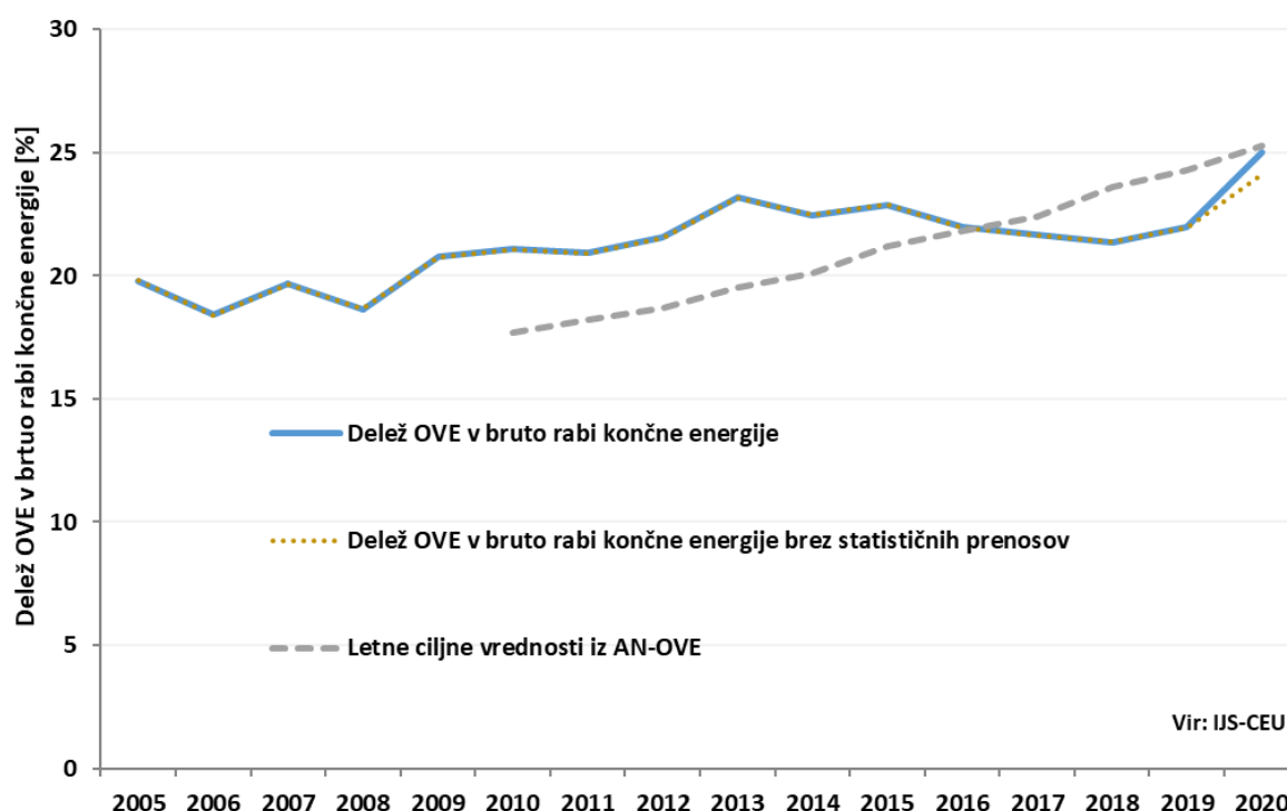
Slika 13: Gibanje skupnega deleža obnovljivih virov energije v bruto rabi končne energije v obdobju 2005–2020 v primerjavi s ciljnim deležem 41 (Vir: IJS-CEU)
