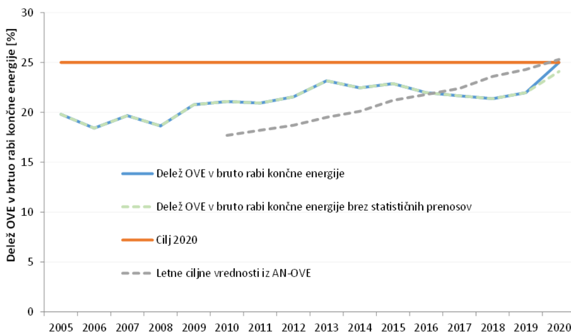
Slika 25: Gibanje deleža OVE v bruto rabi končne energije glede na cilj za leto 2020 in letne projekcijske vrednosti iz AN OVE (Vir: SURS, IJS-CEU)
