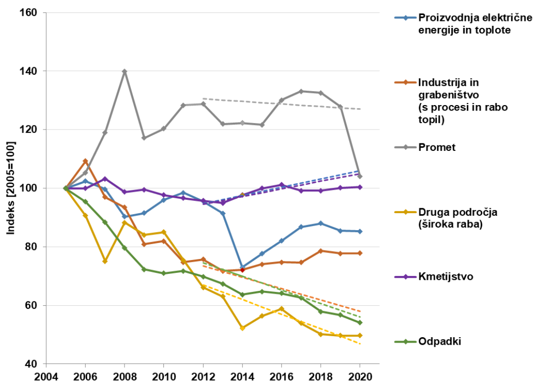
Slika 22: Gibanje emisij neETS po sektorjih v obdobju 2005–2020 v primerjavi s projekcijami za leto 2020 in linearno potjo do ciljev v obdobju 2012–2020 (črtkane črte) (Vir: IJS-CEU)
